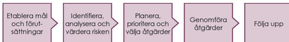
Figur 2. Riskhanteringsprocessen.
