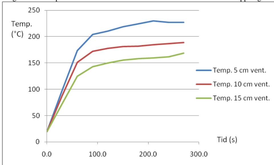
Diagram 10. Temperatur vid värmedetektionskabeln vid de olika ventilationsöppningarna
