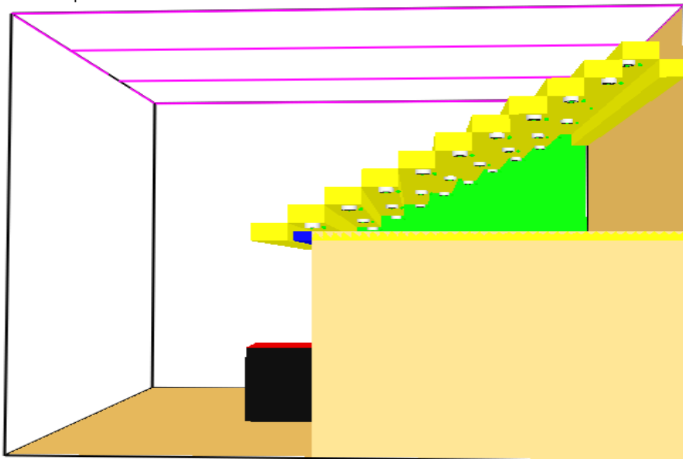
Figur 7. Skolfasaden sedd bakifrån. På den här bilden syns tydligt de optiska rökdetektorernas placeringar samt temperaturmätarna vid varje optisk rökdetektor. Längst till vänster återfinns rökdetektorerna nr 21 (nederst, 5 cm ovan ventilationsöppningen) till nr 30 (överst, taknocken). I centrum återfinns nr 11 (nederst, 5 cm ovan ventilationsöppningen) till nr 20 (överst, taknocken). Längst till höger, närmast betongväggen, återfinns nr 1 (nederst, 5 cm ovan ventilationsöppningen) till nr 10 (överst, taknocken).
