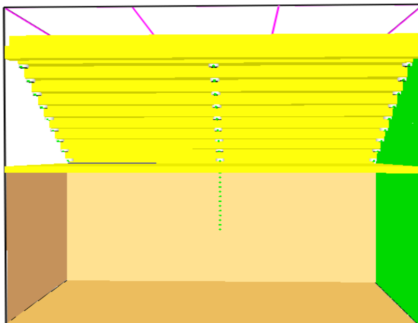
Figur 7. Skolfasaden sedd bakifrån. På den här bilden syns tydligt de optiska rökdetektorernas placeringar samt temperaturmätarna vid varje optisk rökdetektor. Längst till vänster återfinns rökdetektorerna nr 21 (nederst, 5 cm ovan ventilationsöppningen) till nr 30 (överst, taknocken). I centrum återfinns nr 11 (nederst, 5 cm ovan ventilationsöppningen) till nr 20 (överst, taknocken). Längst till höger, närmast betongväggen, återfinns nr 1 (nederst, 5 cm ovan ventilationsöppningen) till nr 10 (överst, taknocken).
