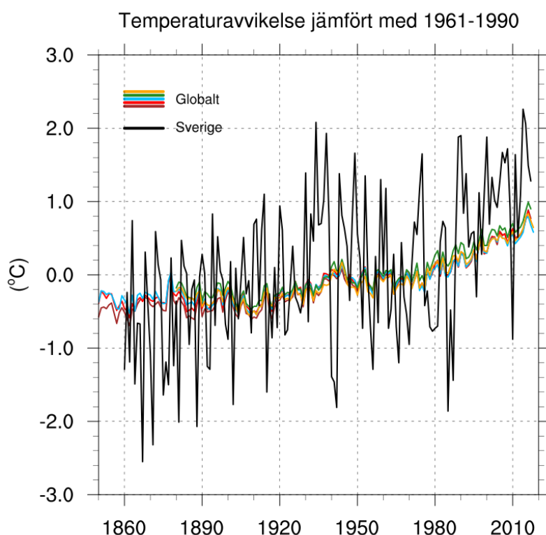
Fig. 4 Temperaturavvikelse jämfört med medelvärdet för perioden 1961-1990 för den globala årsmedeltemperaturen (färgade linjer) och årsmedeltemperaturen i Sverige (svart linje). Variationen mellan år är betydligt större i Sverige än globalt vilket gör att uppvärmningstrenden är svårare att uppfatta.
