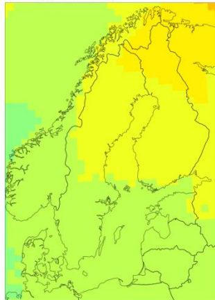
e) RCP 4,5 2071-2100
