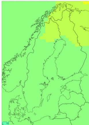
d) RCP 2,6 2071-2100
