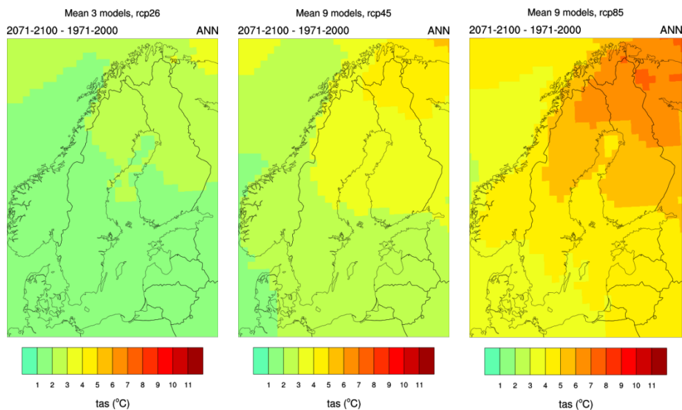
Figur 5 Förändring i årsmedeltemperatur (°C) jämfört med 1971-2000 enligt RCP 8,5 vid a) 2011-2040, b) 2041-2070, c) 2071-2100. Förändring i årsmedeltemperatur 2071-2100 jämfört med 1971-2000 enligt d) RCP 2,6, e) RCP 4,5, f) RCP 8,5 [8] .
