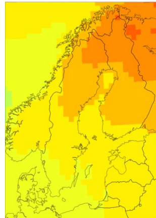
f) RCP 8,5 2071-2100
