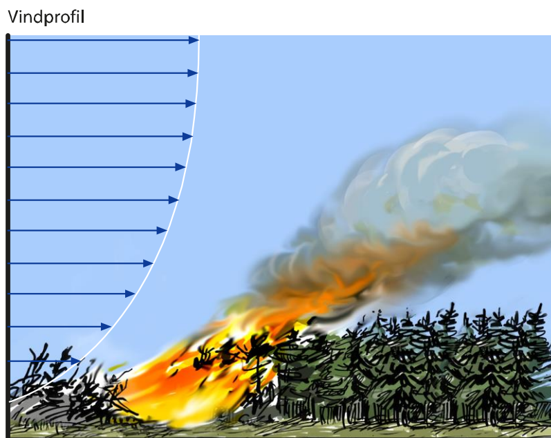
Figur 2. Vindburen toppbrand kan uppkomma när vindstyrkan ökar och brandgaser från brinnande träd antänder angränsande trädtoppar.
