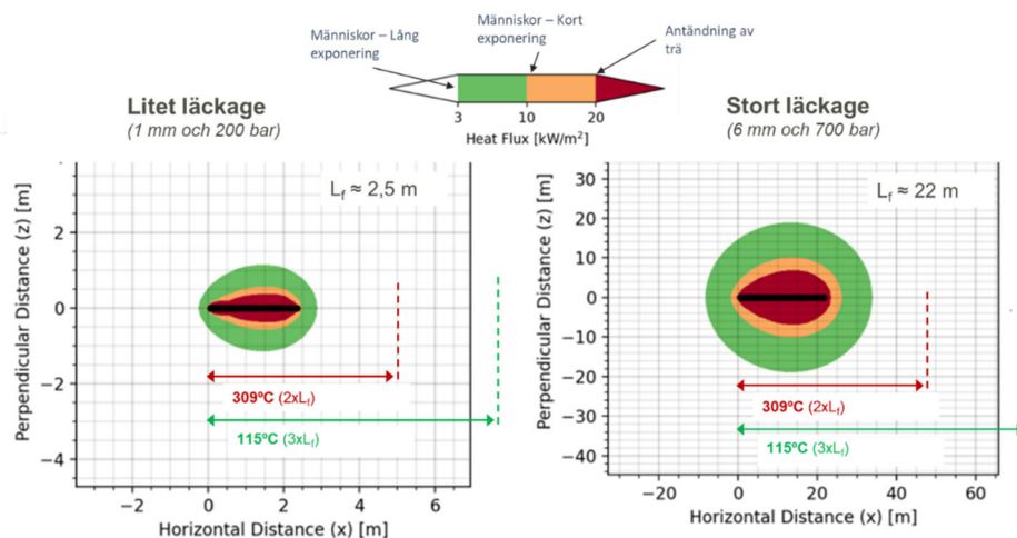
Figur 7. Jämförelse mellan avstånd för skadliga förhållanden gällande strålning samt temperatur där 309°C ger tredje gradens brännskada efter 20 sekunder och 115°C ger smärta efter 5 min (Molkov, 2012). Svart linje motsvarar flamlängden.
