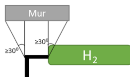
Figur 16. Illustration av barriärens minsta bredd.
