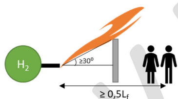
Figur 14. Barriärens minsta höjd och dess påverkan på avstånd till människor.
