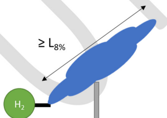
Figur 15. Barriärens minsta höjd och dess påverkan på avstånd för icke antända utsläpp.
