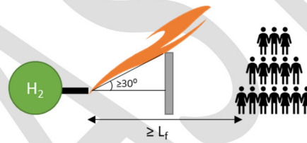
Figur 14. Barriärens minsta höjd och dess påverkan på avstånd till människor.
