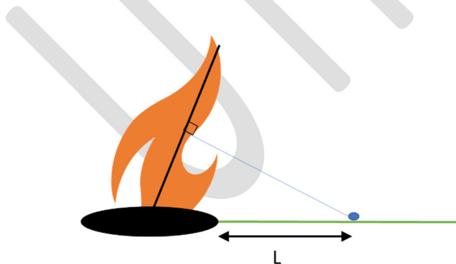
Figur 11. Strålning från vindpåverkad flamma.
