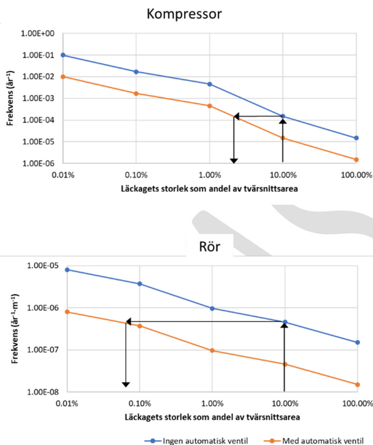
Figur 9. Påverkan av automatiska avstängningsventiler på dimensionerande skadefall för rör respektive kompressor.
