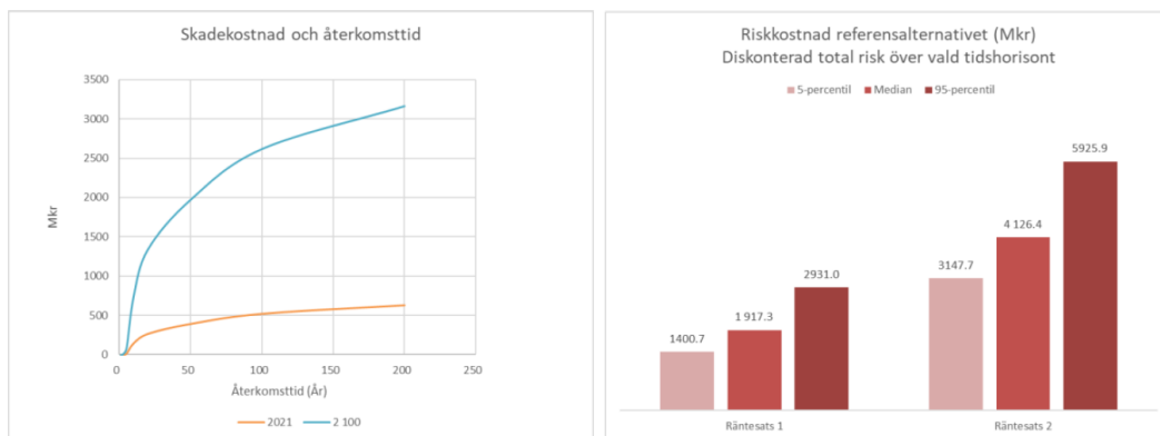
Figur 7. Skadekostnad och återkomsttid samt beräknad total riskkostnad till följd av översvämning från stigande nivåer i havet under tidsperioden år 2021–2100 beräknad med Räntesats 1 (3,5 %) och Räntesats 2 (1,4 %) för område Syd.
