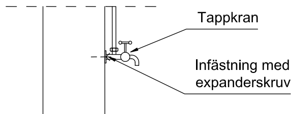
Figur T19-102a. Sektion genom tappställe.
