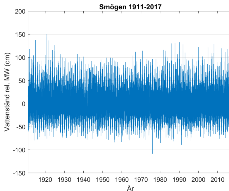
Figur 2. Havsvattenstånd i cm relativt medelvattenytan vid Smögen 1911-2017.
